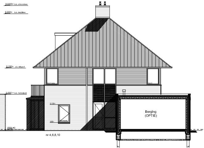
Rechterzijgevel
