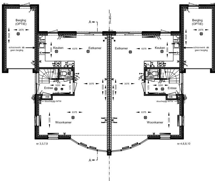
Begane grond
