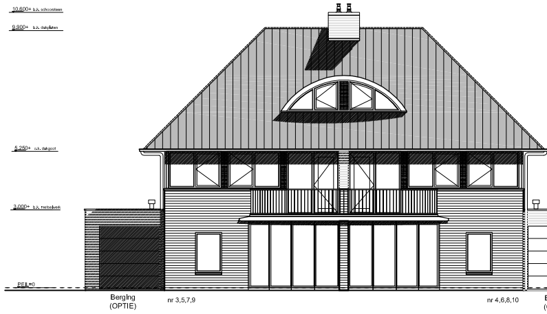
Voorgevel
