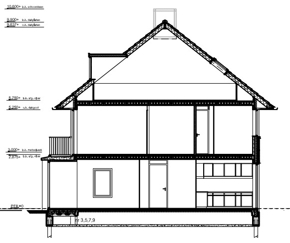
Doorsnede AA
